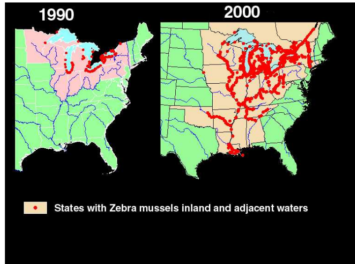
Figura 2: La expansión de la plaga en Norteamérica.
