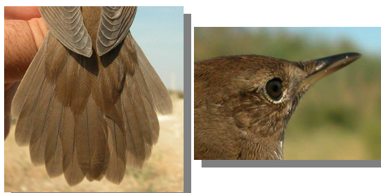
Buscarla unicolor. Diseño de la cola y ausencia de cerdas en la boca.
